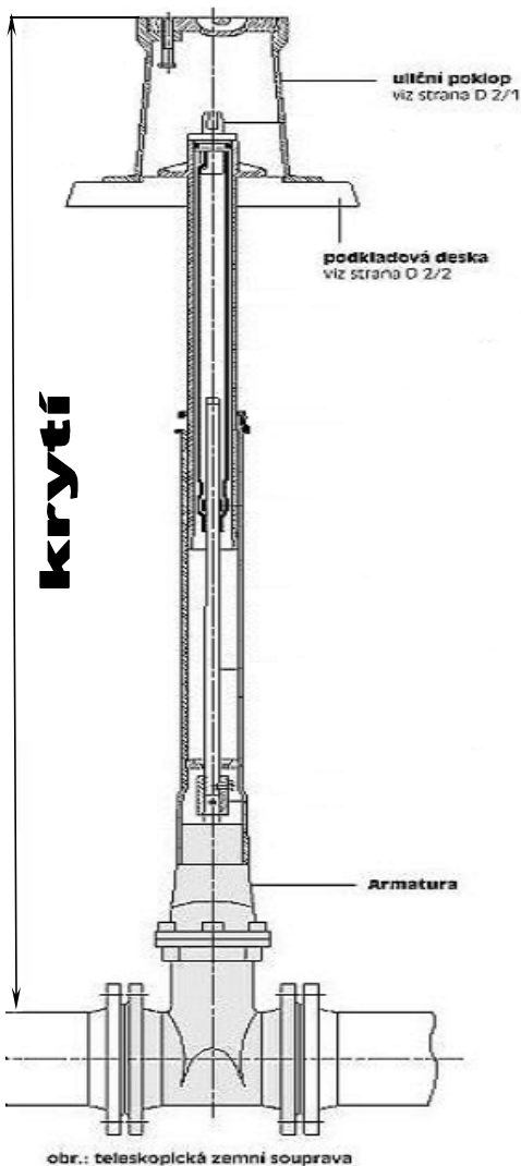
obr.: teleskopická zemní souprava
